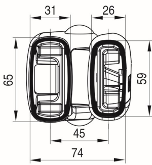
projections de 160 à 310cm BRAS DOUBLE CABLE GAINÉ
